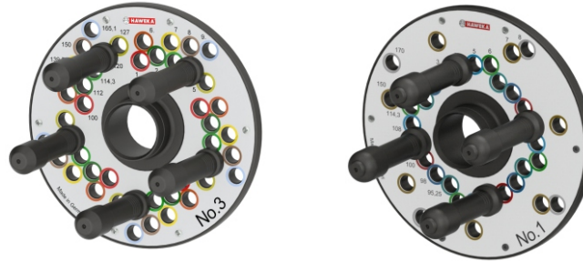
VAS 6243 VAS 6242 ASE 422 062 00 000 ASE 422 061 00 000
